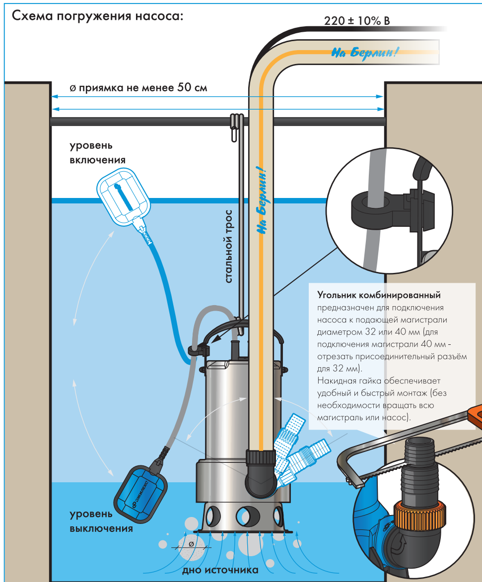
Рисунок 3 (на примере изображен насос погружной «ФЕКАЛЬНИК» 150/7Н).
